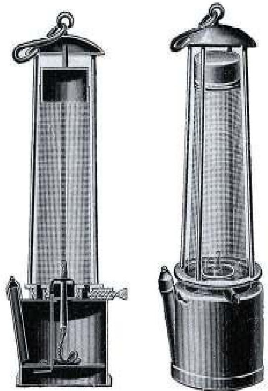
ආරක්‍ෂක ලාම්පුව
