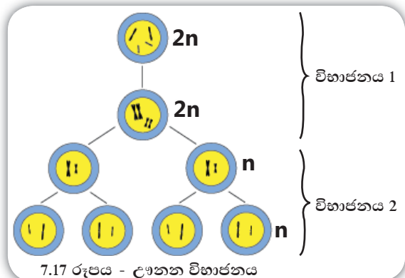
7.17 රූපය - ඌනත විභාජනය
