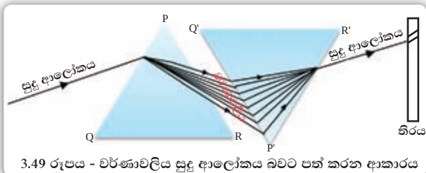
3.49 රූපය - වර්ණාවලිය සුදු ආලෝකය බවට පත් කරන ආකාරය
