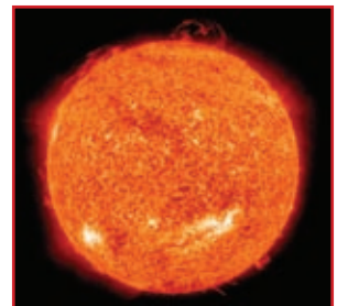
4.3 රූපය - සූර්යයා
