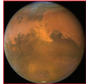
4.4 රූපය - බුධ
